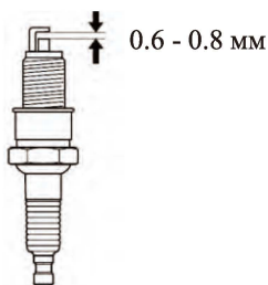
Рисунок 6. Межэлектродный зазор свечи зажигания.
