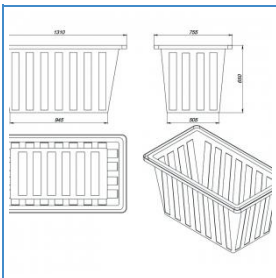
Ванна К 400 литров Артикул: 132.0400.601.0 ВхШхД: 650x755x1310
