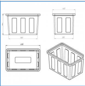
Ванна К 90 литров Артикул: 132.0090.601.0 ВхШхД: 425x460x690
