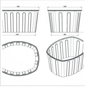
Ванна 1000 литров Артикул: 131.1000.601.0 ВхШхД: 800x1250x1550
