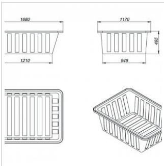
Ванна К 600 литров Артикул: 132.0600.601.0 ВхШхД: 495x1170x1680
