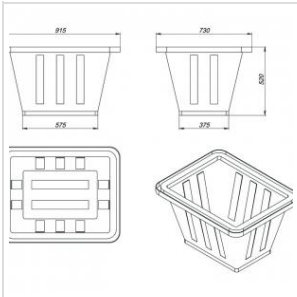
Ванна К 200 литров Артикул: 132.0200.601.0 ВхШхД: 520x730x915
