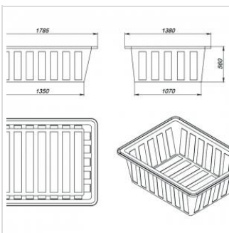
Ванна К 900 литров Артикул: 132.0900.601.0 ВхШхД: 560x1380x1785
